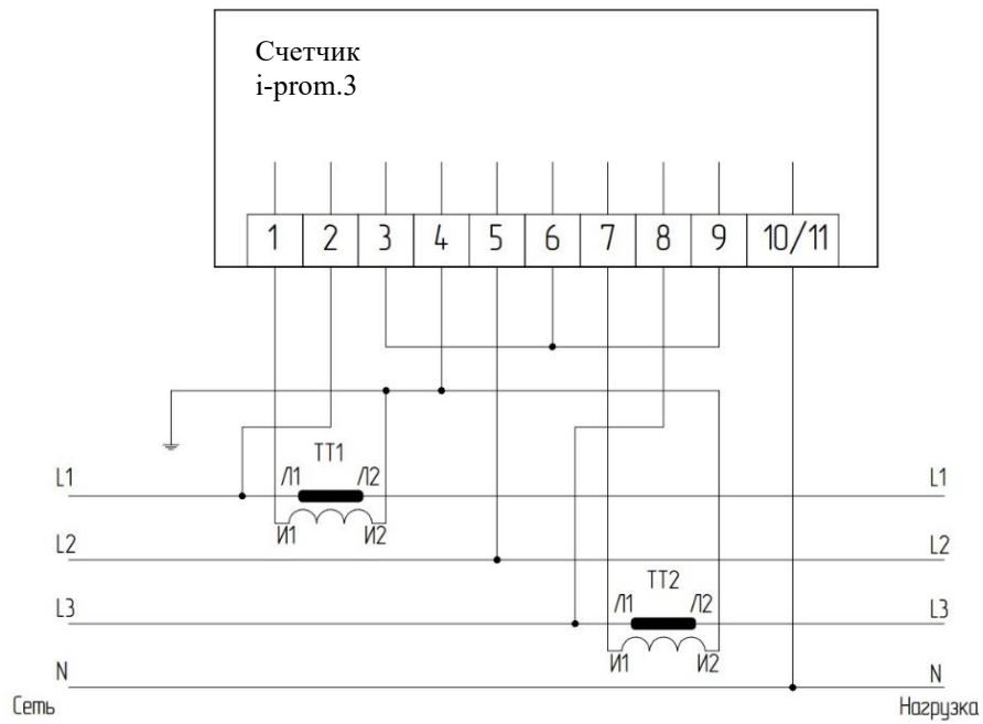
Рисунок В.3 – Схема подключения счетчика электрической энергии трехфазного многофункционального i-пром.3 трансформаторного включения через два трансформатора тока
