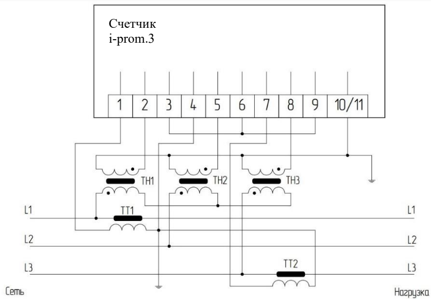
Рисунок В.5 – Схема подключения счетчика электрической энергии трехфазного многофункционального i-пром.3 трансформаторного включения через три трансформатора напряжения и два трансформатора тока
