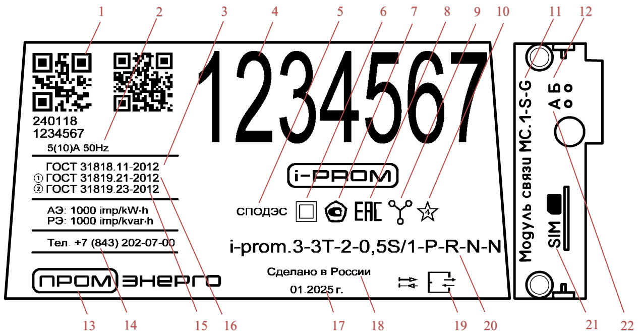
Рисунок 4.5 - Маркировка счётчиков электрической энергии трехфазных многофункциональных i-prom.3 в корпусе «S» – Split
