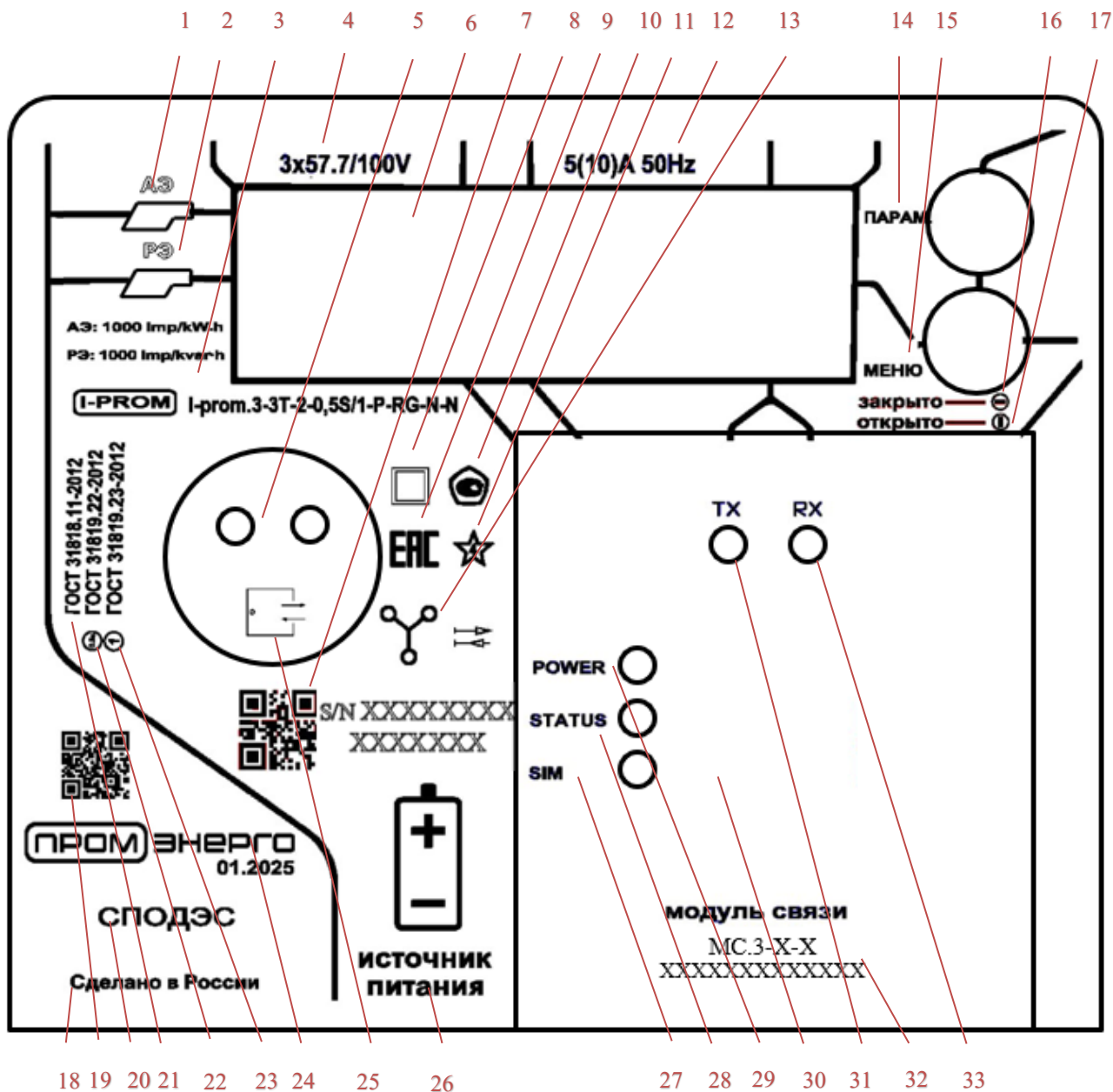
Рисунок 4.3 - Маркировка счётчиков электрической энергии трехфазных многофункциональных i-prom.3 трансформаторного косвенного включения
