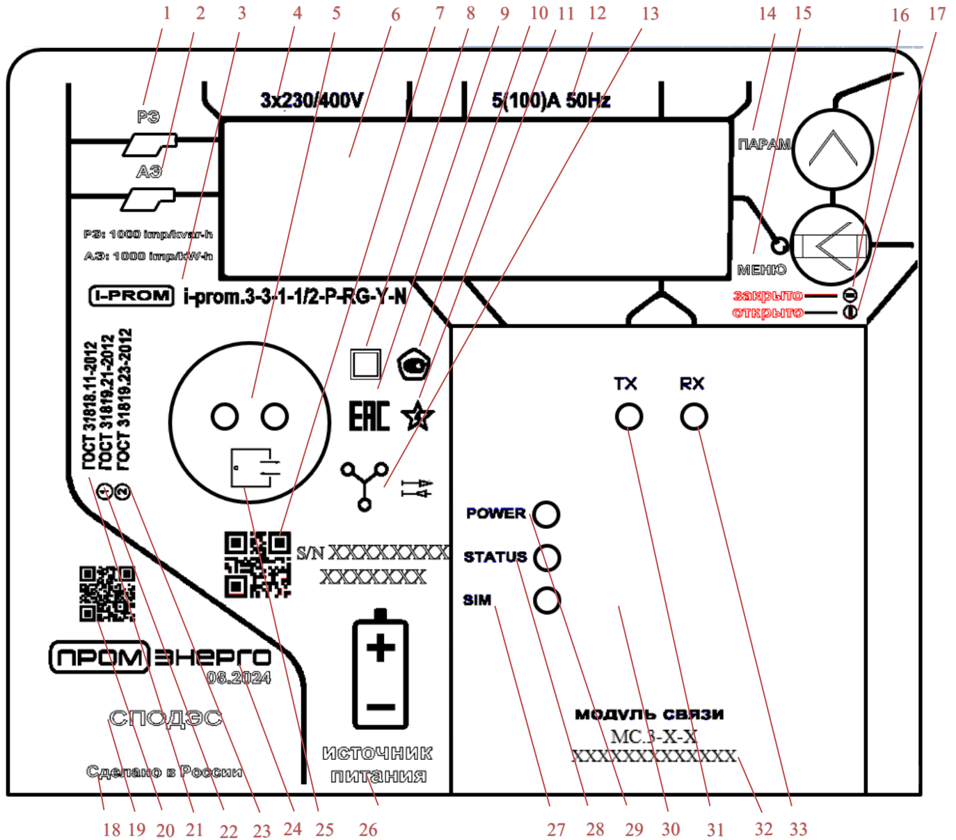
Рисунок 4.2 - Маркировка счётчиков электрической энергии трехфазных многофункциональных i-prom.3 прямого включения
