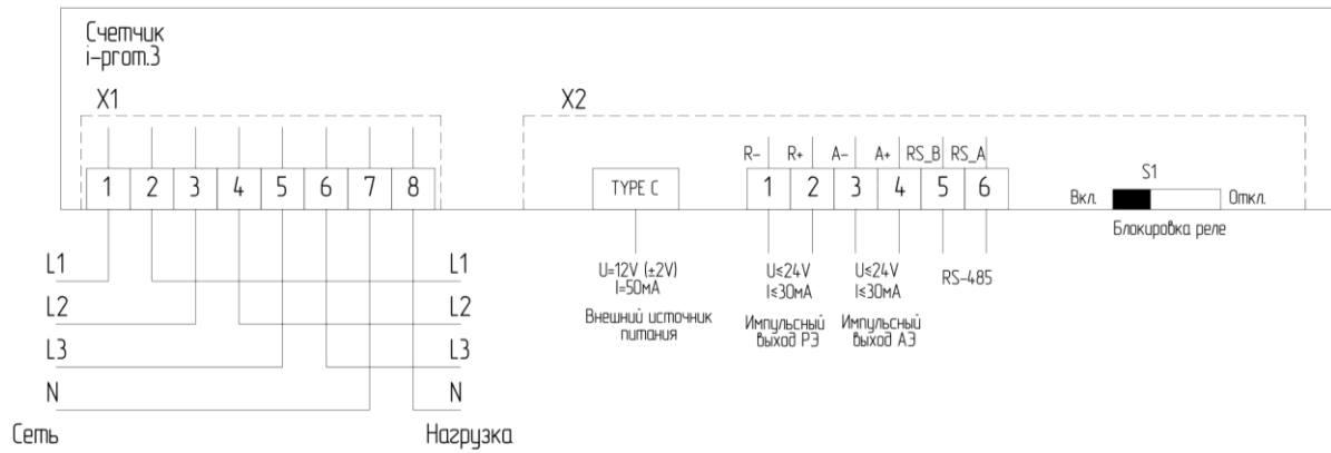
Рисунок В.16 – Схема подключения счетчика электрической энергии трехфазного многофункционального i-prom.3 в корпусе «S» – Split
