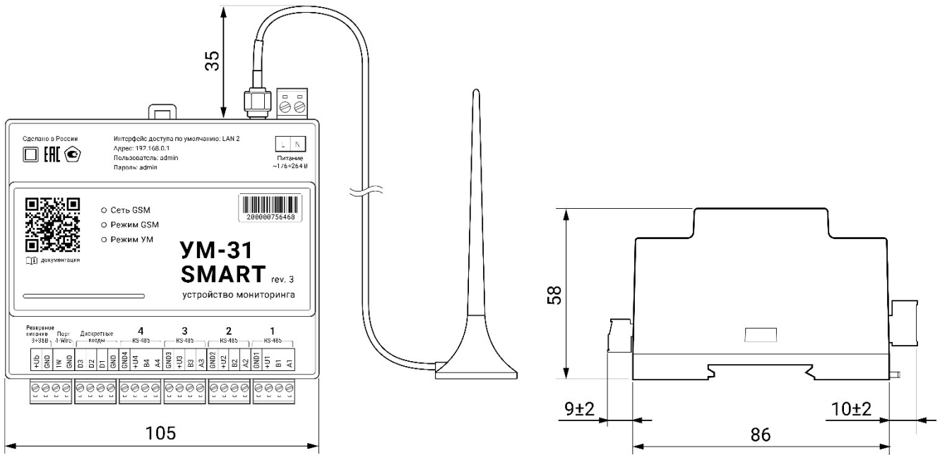
Рисунок 1 – Габаритные размеры УМ
