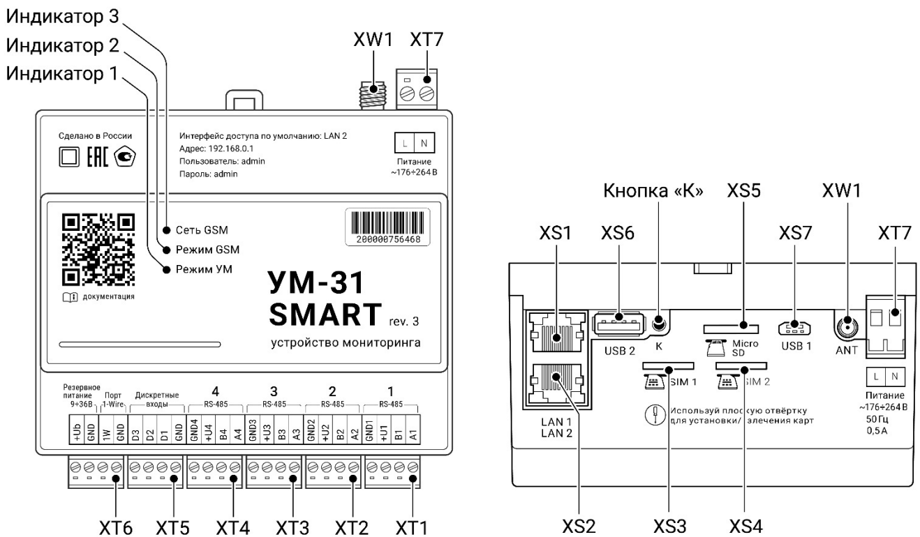
Рисунок 3 – Расположение разъёмных соединителей, индикаторов и кнопок
